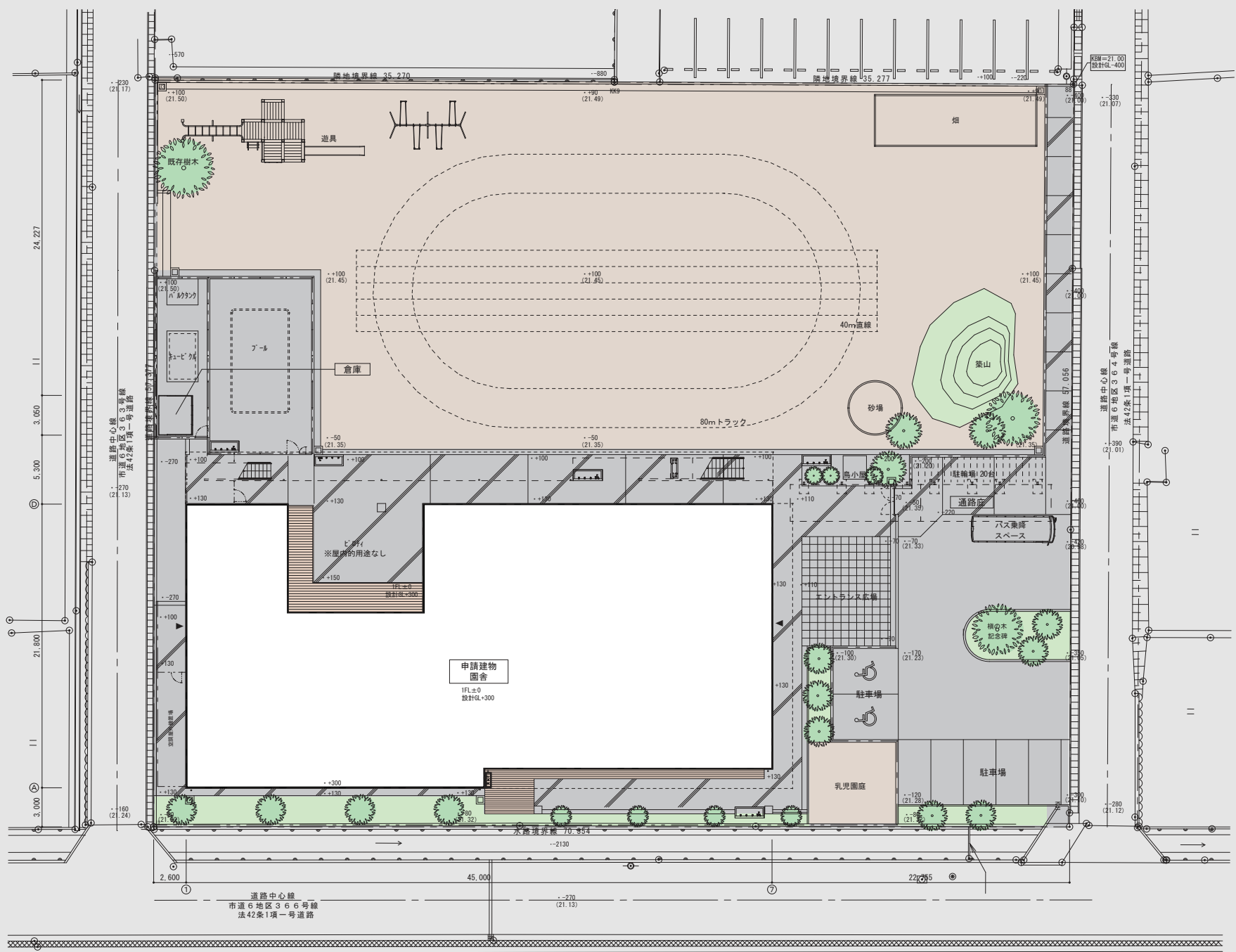
配置図
